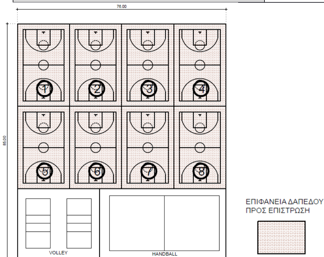
Εικόνα 1: Κάτοψη των υπαίθριων γηπέδων καλαθοσφαίρισης του Ποσειδωνίου Αθλητικού Κέντρου προς επίστρωση.
