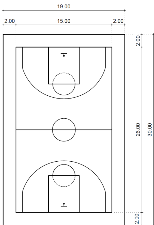
Εικόνα 2: Τυπικό υπαίθριο γήπεδο καλαθοσφαίρισης στο Ποσειδώνιο Αθλητικό Κέντρο Θεσσαλονίκης.
